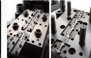
精密微細順送プレス金型
