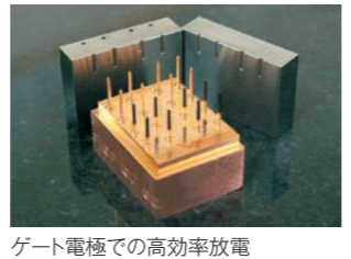
ゲート電極での高効率放電
